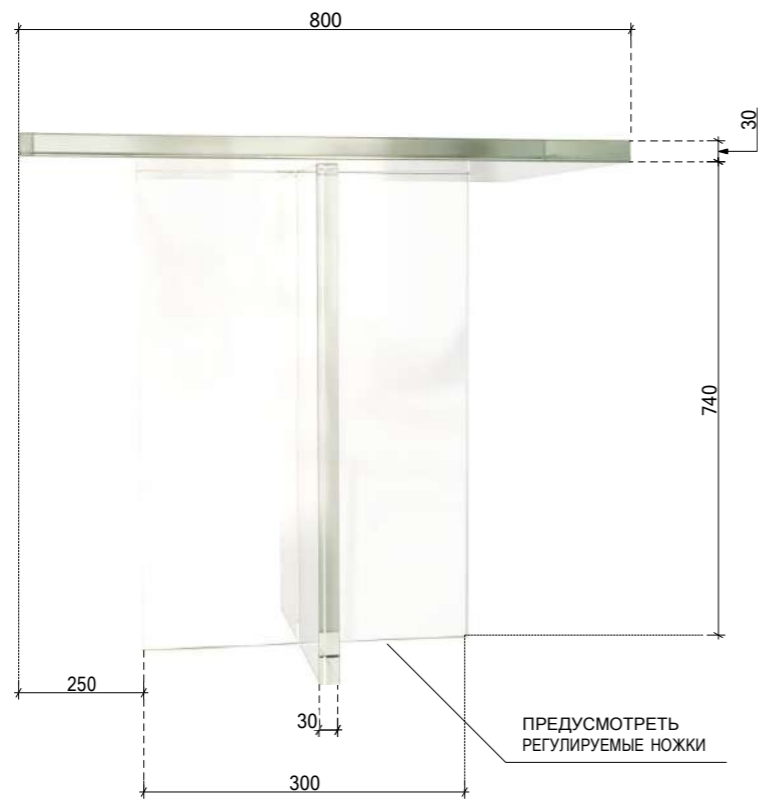
ВИД СПЕРЕДИ
